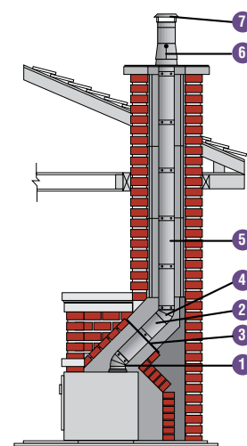
Installation avec déboîtement
